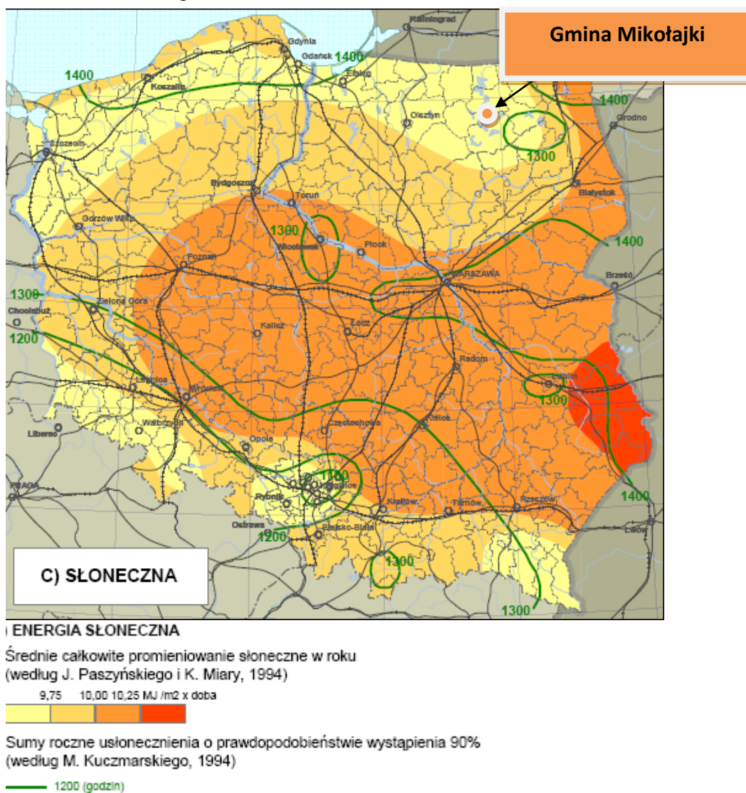
Rys. 3. Średnie całkowite promieniowanie słoneczne w roku
